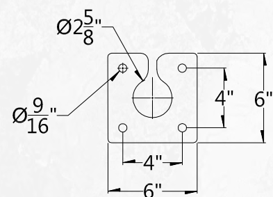
PATRON DE BOULONNAGE DES SUPPORTS
