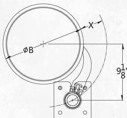
PATRON DE BOULONNAGE DES SUPPORTS
