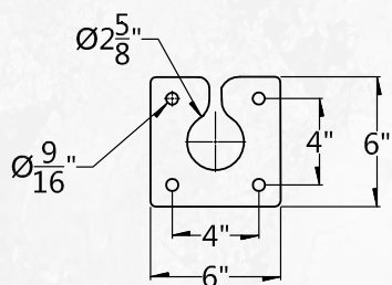
PATRON DE BOULONNAGE DES SUPPORTS
